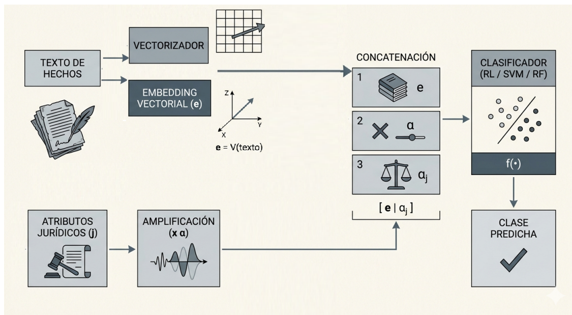
Figura 5.6: Arquitectura del pipeline de clasificación combinado
