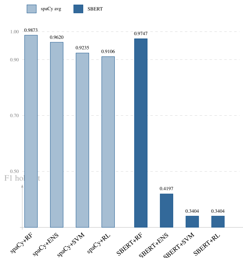
Figura 5.7: F1 ponderado en holdout por combinación de modelo (evaluación sin atributos jurídicos)
